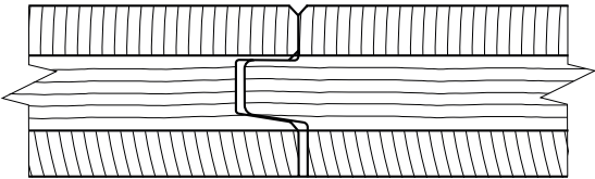
Umlaufend Keil-Nut-Feder Verbindung mit Fase * Nur längsseitig mit Nut + Feder möglich
